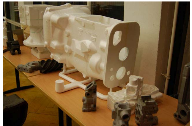
Nach dem lost foam Verfahren hergestellte Gussstücke und Modelle
